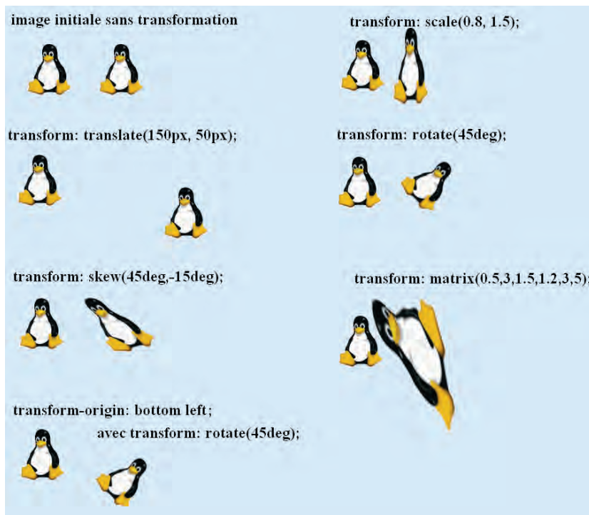
FIGURE B-7 Quelques transformations géométriques à deux dimensions en CSS 3, affichées par le navigateur Chrome.
